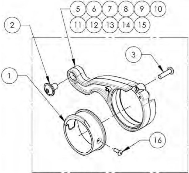
ACTUAL ASSEMBLY
